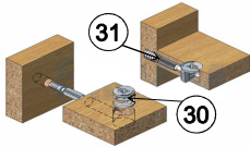
Эксцентриковая стяжка
